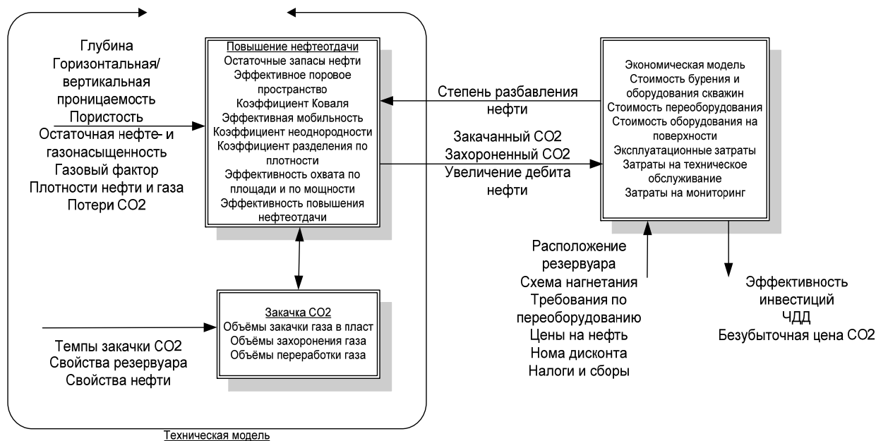
Рис. 1 – Принципиальная схема технико-экономической модели закачки \text{CO}_2 в нефтяное месторождение [4]
